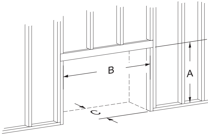
Ouverture brute pour installation au niveau du sol
