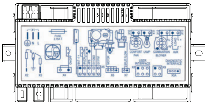
Dessus du module récepteur Figure 26
