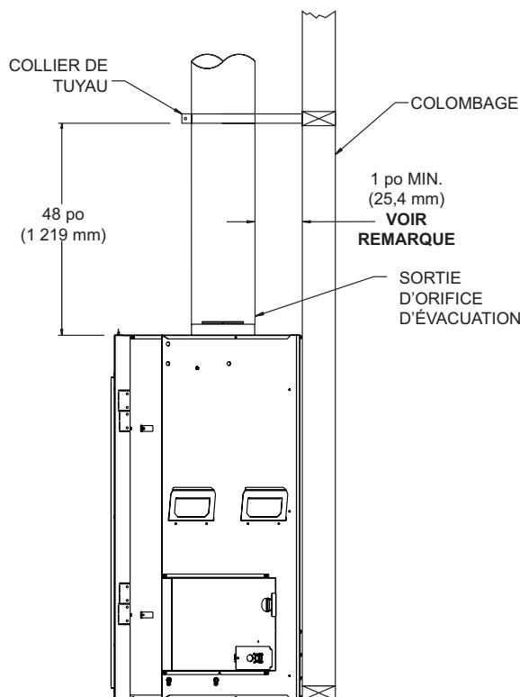
Installation de coupe-feu - Figure 39
