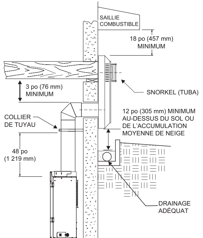
INSTALLATION TYPE EN SOUS-SOL MODÈLE GÉNÉRIQUE ILLUSTRÉ
