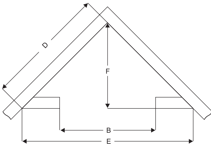
Ouverture brute pour installation en coin
